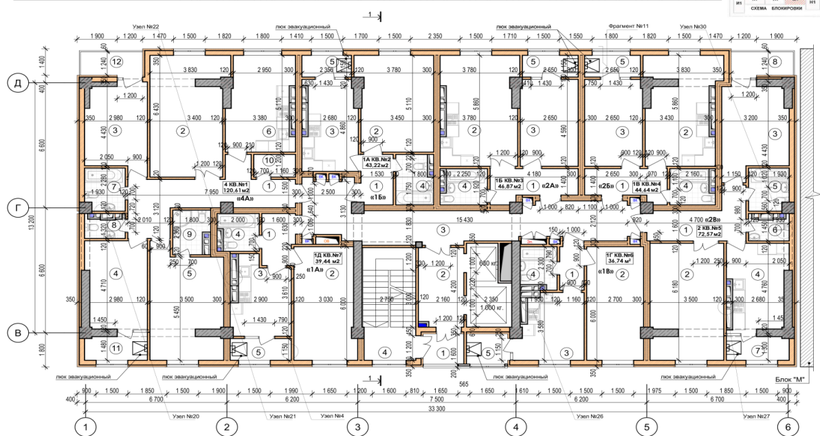
План стен типового этажа на отм. +3.500; +6.650; +9.800; +12.950; +16.100; +19.250; +22.400; +25.550; +28.700; +31.850; +35.000; +38.150. М1:100
