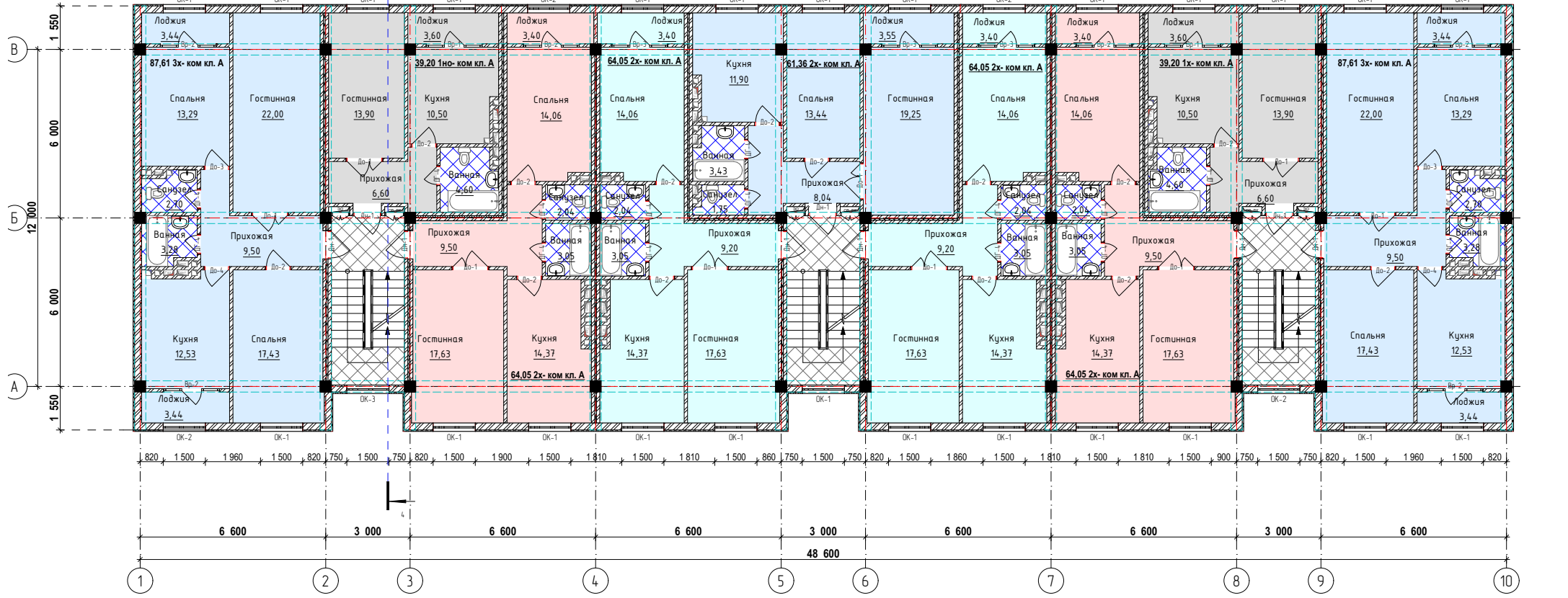
План с 2 - го по 5 - ый этаж, Блок - 1,2,3,4,5
