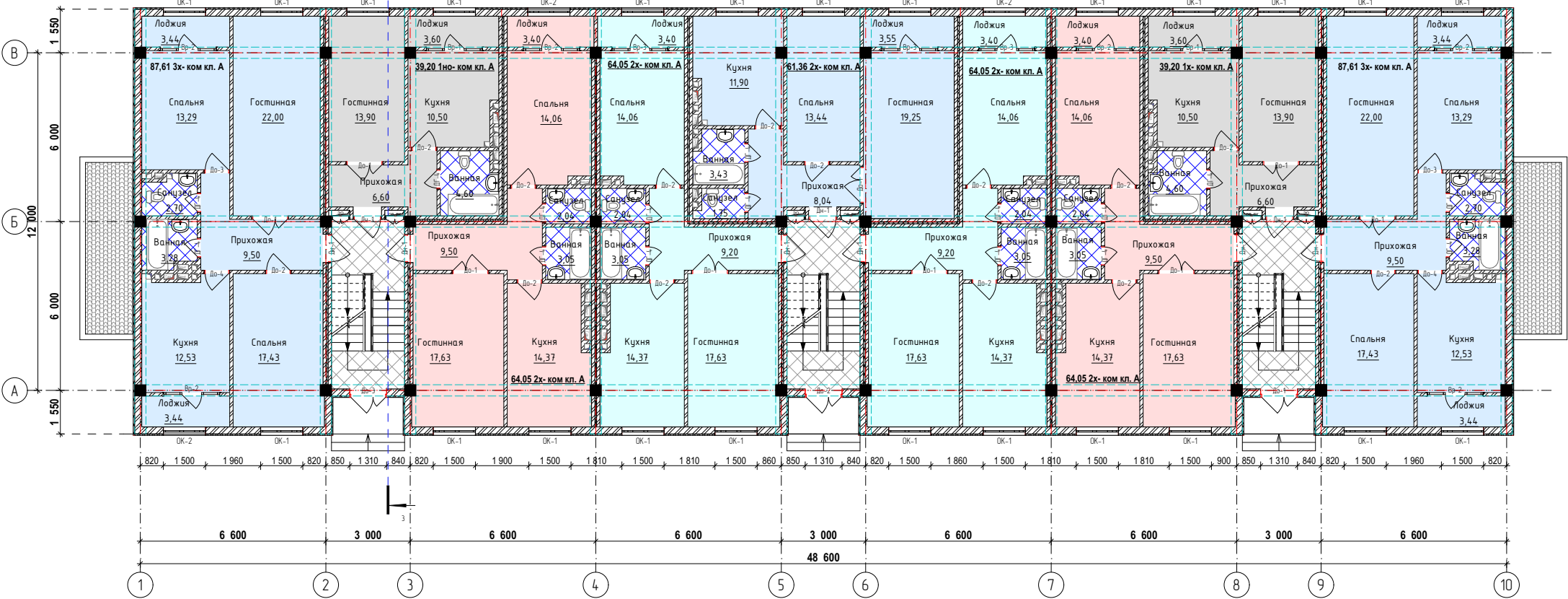
План 1 - го этажа, Блок - 1,2,3,4,5
